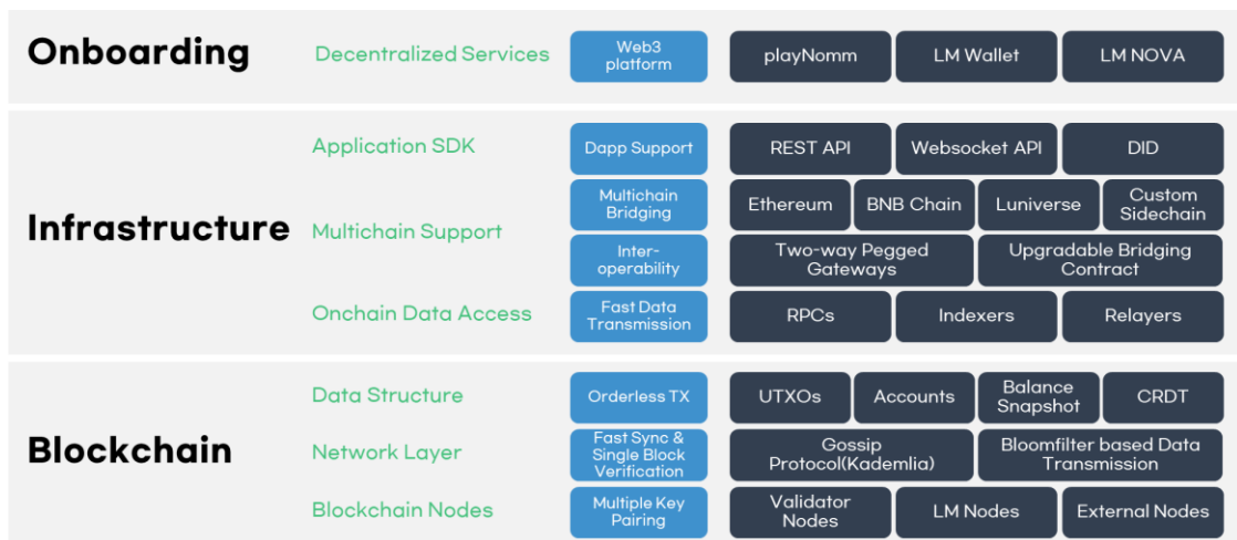
[레저메타버스 블록체인의 구조]
